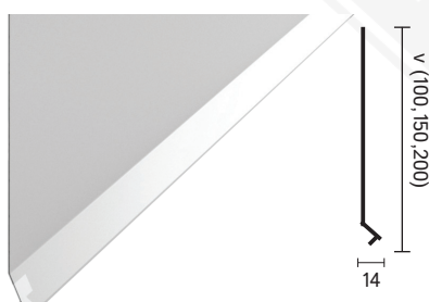
Plech - STONE / RT Materiál: Al
