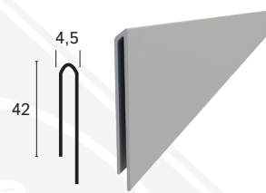
Nadstavec – RT/30 mm Materiál: Al
