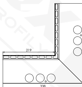
Kút – RT/30 mm Materiál: Al
